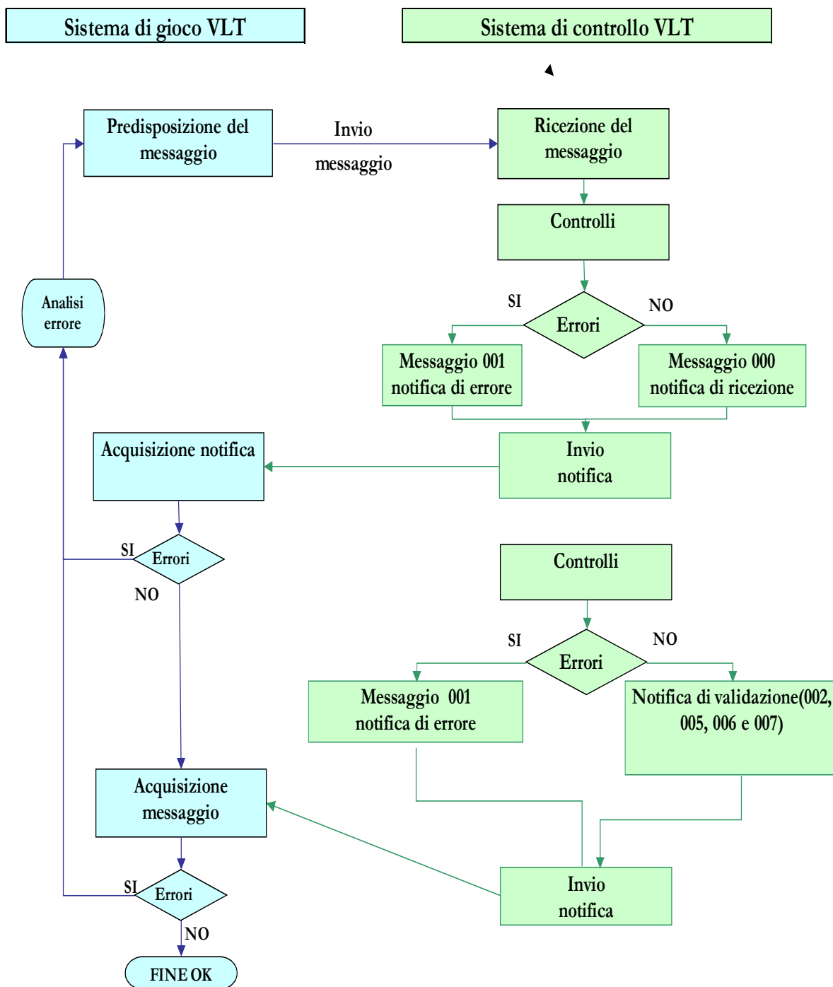
Figura 1 Flusso di comunicazione sistema di gioco VLT - sistema di controllo VLT
