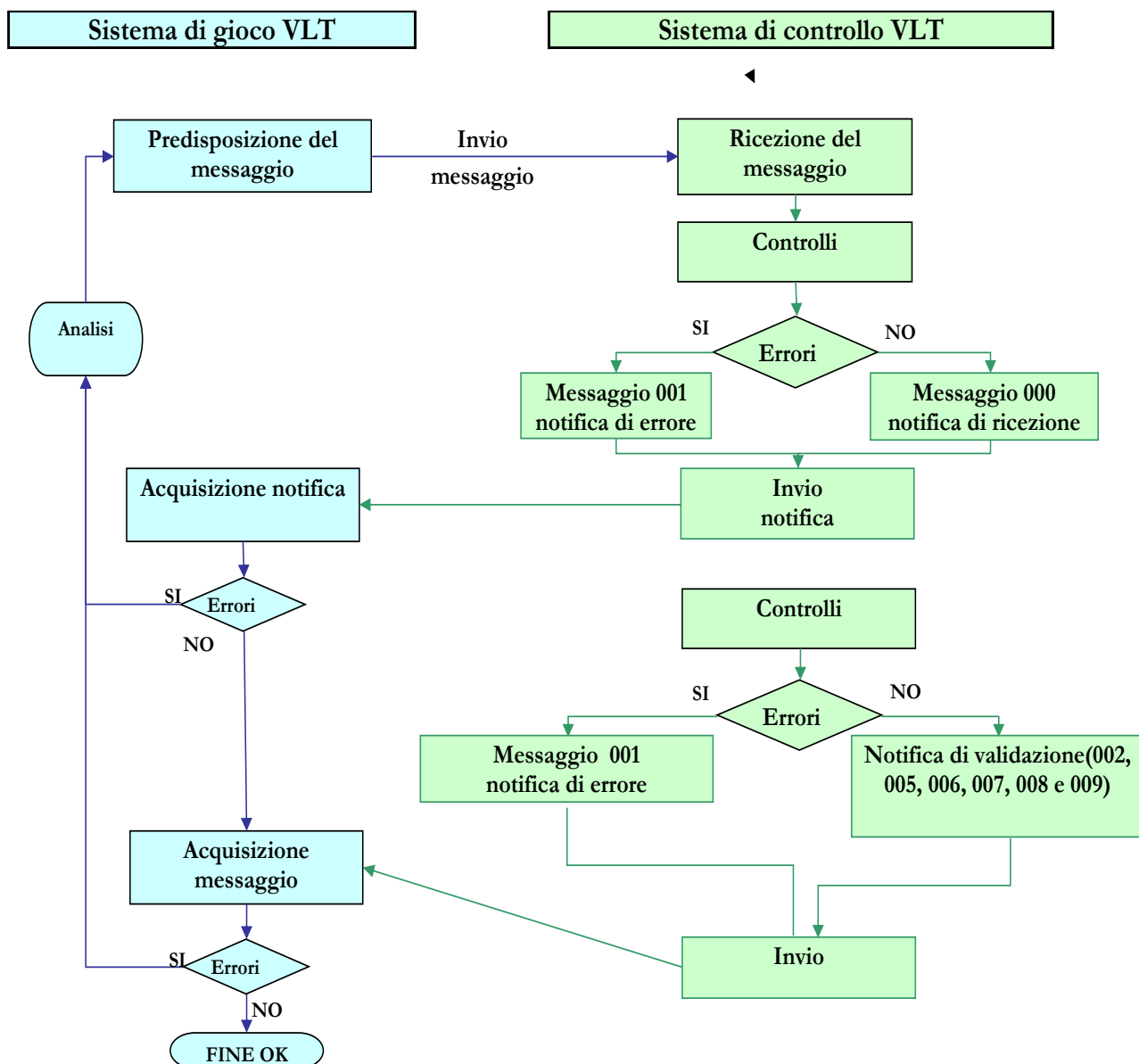
Figura 1 Flusso di comunicazione sistema di gioco VLT - sistema di controllo VLT
