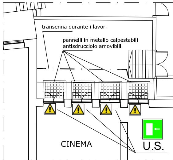
PIANTA QUOTA +0.00
