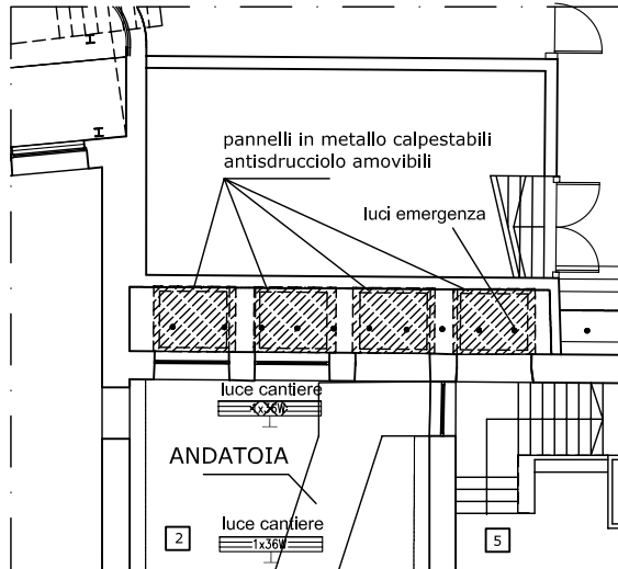
PIANTA QUOTA -1.80
